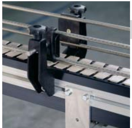
Guide laterali standard con regolazione della larghezza
